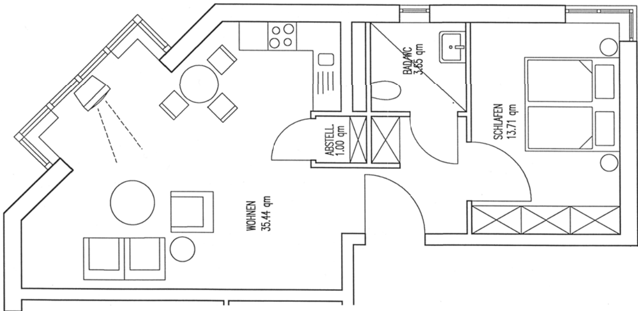
Grundriss Seniorenwohnen, Typ D
